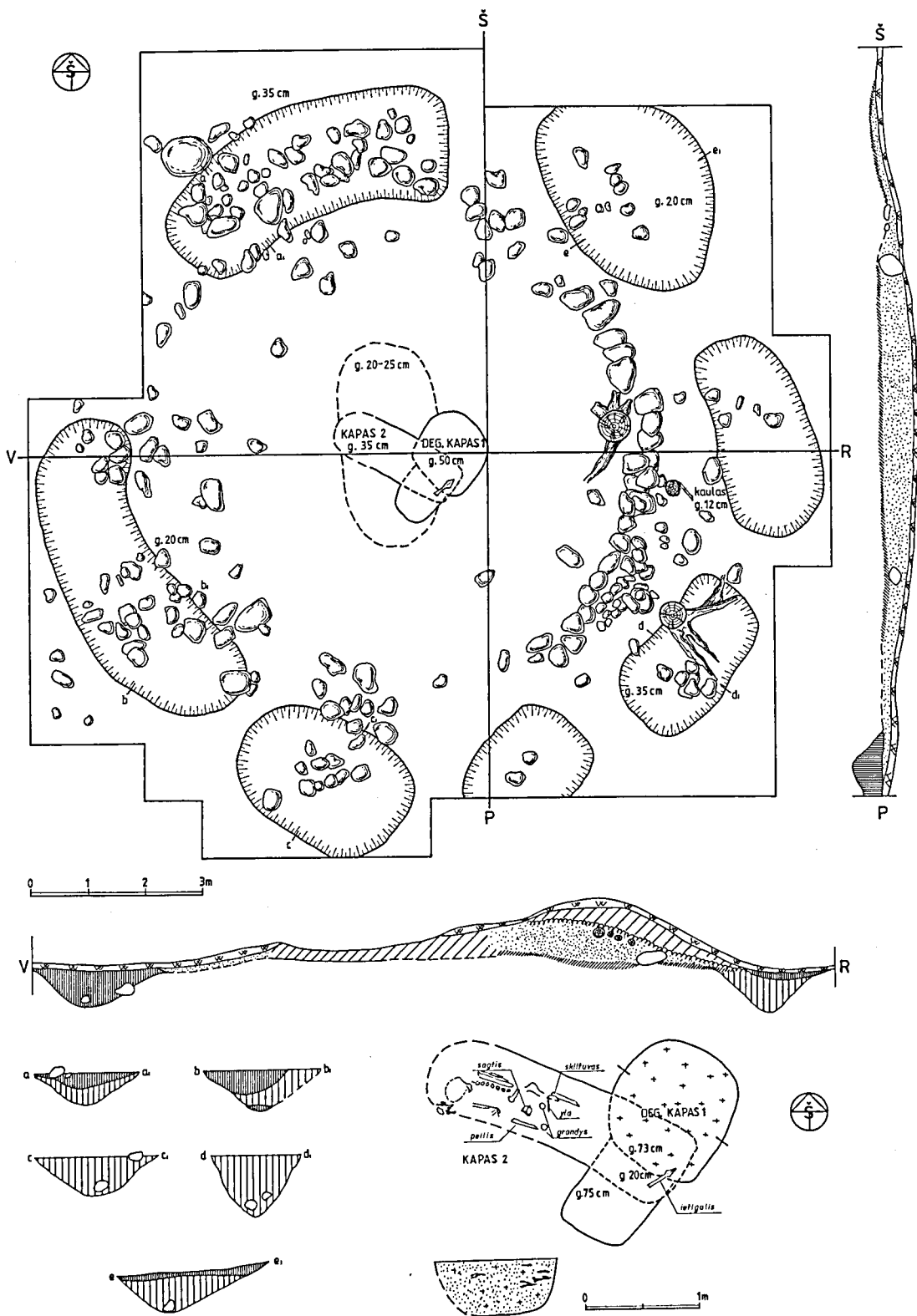
26 pav. Pilkapio 4 planas. R. Abramauskienės, V. Kliugaitės brėž. Fig. 26. Plan of barrow 4.
