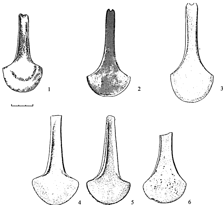
5 pav. Atkraštiniai kirviai: Rytų Pabaltijo tipo kirvis iš Lietuvos (1); Langquaido II tipo kirviai (2, 3); Rytų Pabaltijo tipo kirviai iš Smørumovre (Danija) lobio (4–5), (pagal LAA I, pav. 18, 9; Abels 1972, Taf. 21, Nr. 289; Moora 1932, Abb. 14, 2; Aner, Kersten 1973, Taf. 63).
