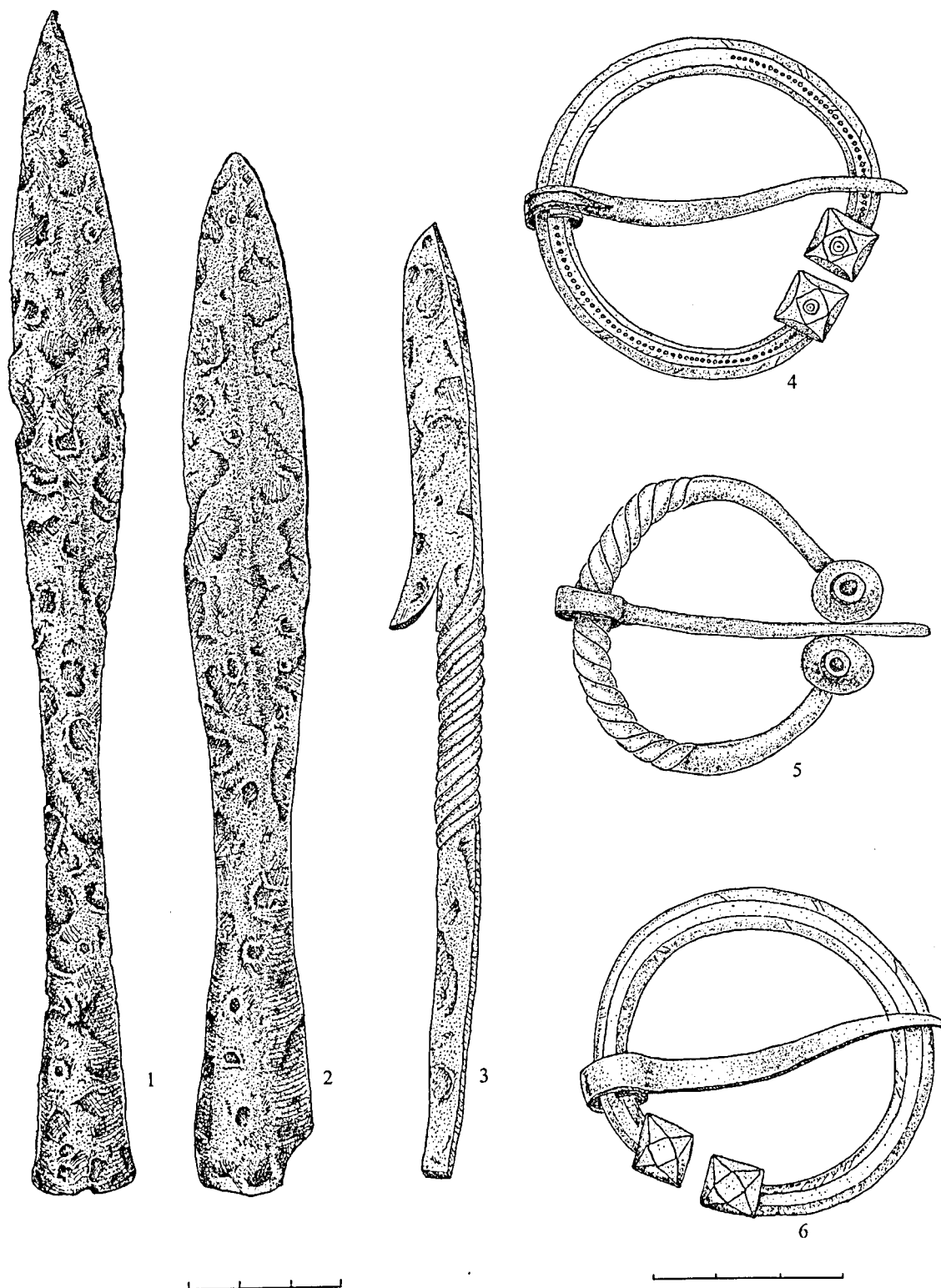
8 pav. Kapų 1, 11, 27 įkapės: 1 – įmovinis karklo lapo formos ictigalis iš k. 1; 2 – įmovinis karklo lapo formos ictigalis iš k. 11; 3 – įtviriamasis ictigalis su užbarzda iš k. 27; 4–6 – pasaginės segės iš k. 1, 27, 11. S. Mikšaitės pieš.
