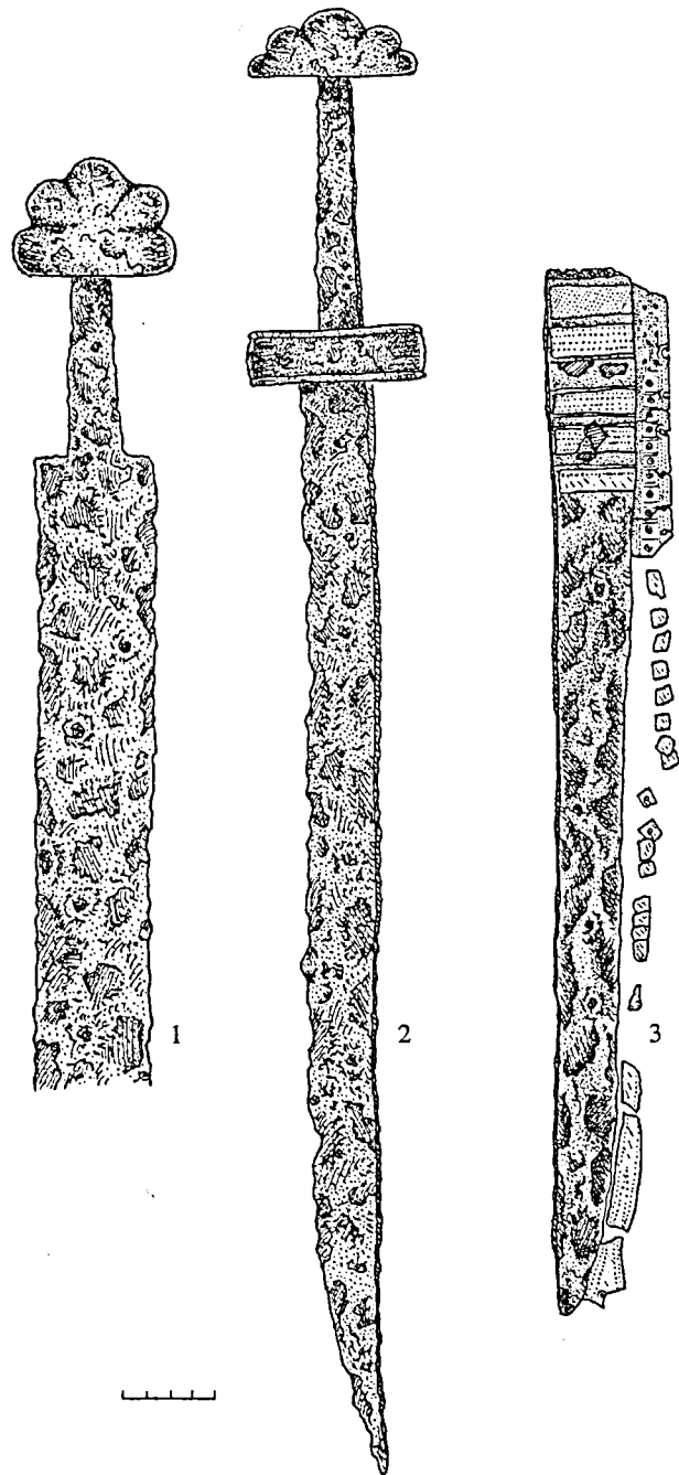
10 pav. Kalavijai ir kovos peilis: 1 – kalavijas iš k. 27; 2 – kalavijas iš k. 145; 3 – siauras ilgas kovos peilis iš k. 18. S. Mikšaitės pieš.
