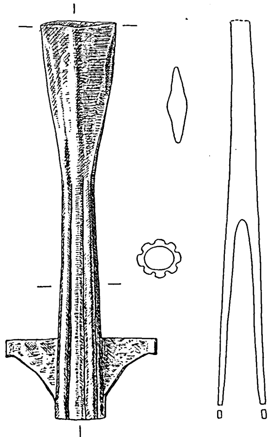
5 pav. Ietigalis su sparneliais (piešė V. Laužadienė).
