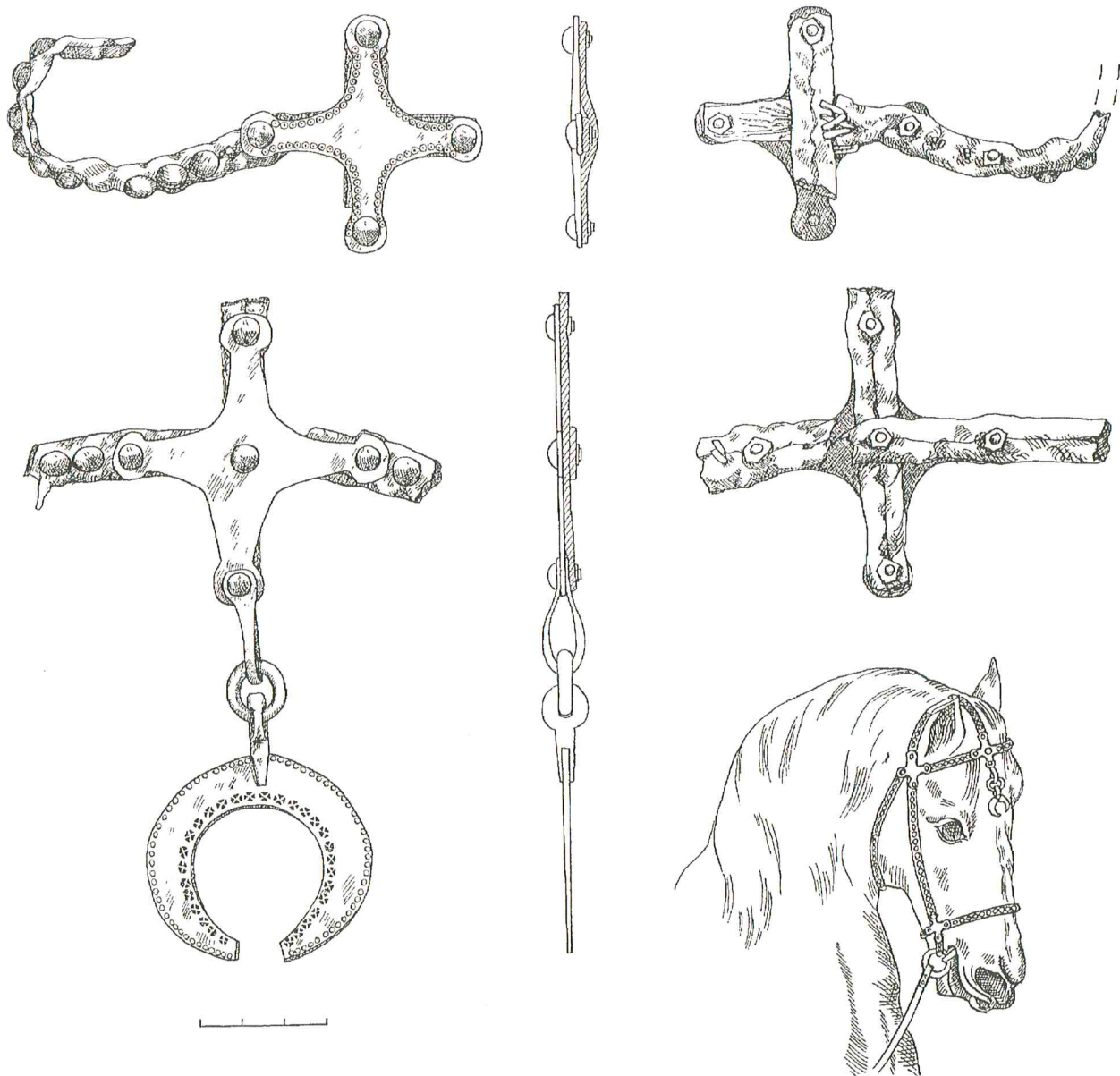
214 pav. Kamanų apkaustai iš vyro kapo Nr. 47
