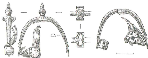
211 pav. Pentinai iš vyro kapo Nr. 47
