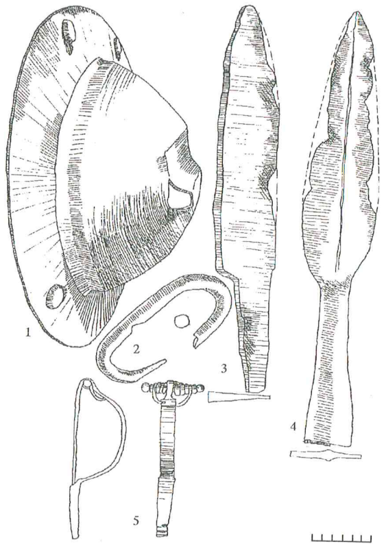
9 p a v. Pilkapio 3(3) radiniai: 1 – skydo umbas, 2 – diržo sagtis, 3 – peilis, 4 – ietigalis, 5 – segė; 1–4 geležis, 5 – žalvaris. Piešė J. Dičmonaitė
