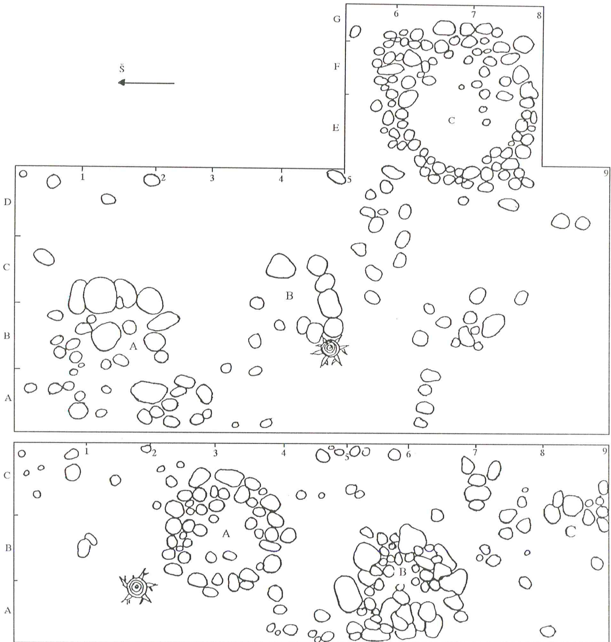
7 p a v . Perkasų III (apačioje) ir IV (viršuje) planai su akmenų vainikais. Piešė A. Ruzienė
