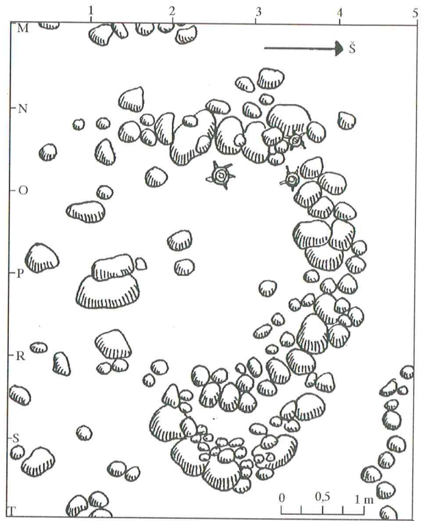
4 p a v. Perkastos II dalis, pilkapio 18(21) akmenų vainikas su pusbėnelio formos priedu. Piešė A. Ruzienė
