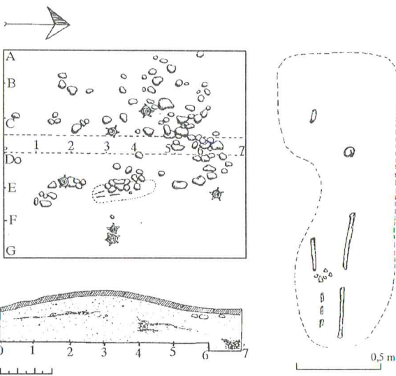
33 p. v. Pilkapis 11(10) ir sampilo pjūvis šiaurės–pietų kryptimi bei griautinio kapo likučiai su žalvariniu žiediniu antsmilkiniu. Piešė A. Ruzienė
