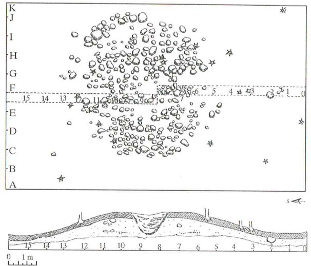
36 p. v. Pilkapio 15(22) akmenų konstrukcija (grindinys ir dalis akmenų vainiko). Piešė A. Ruzienė
