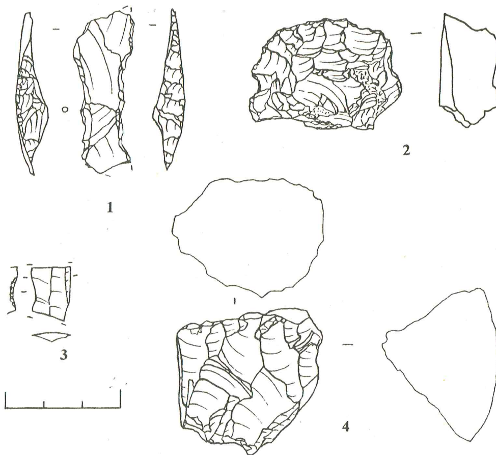
11 pav. Upėtų 2-osios stovyklavietės titnago dirbiniai
