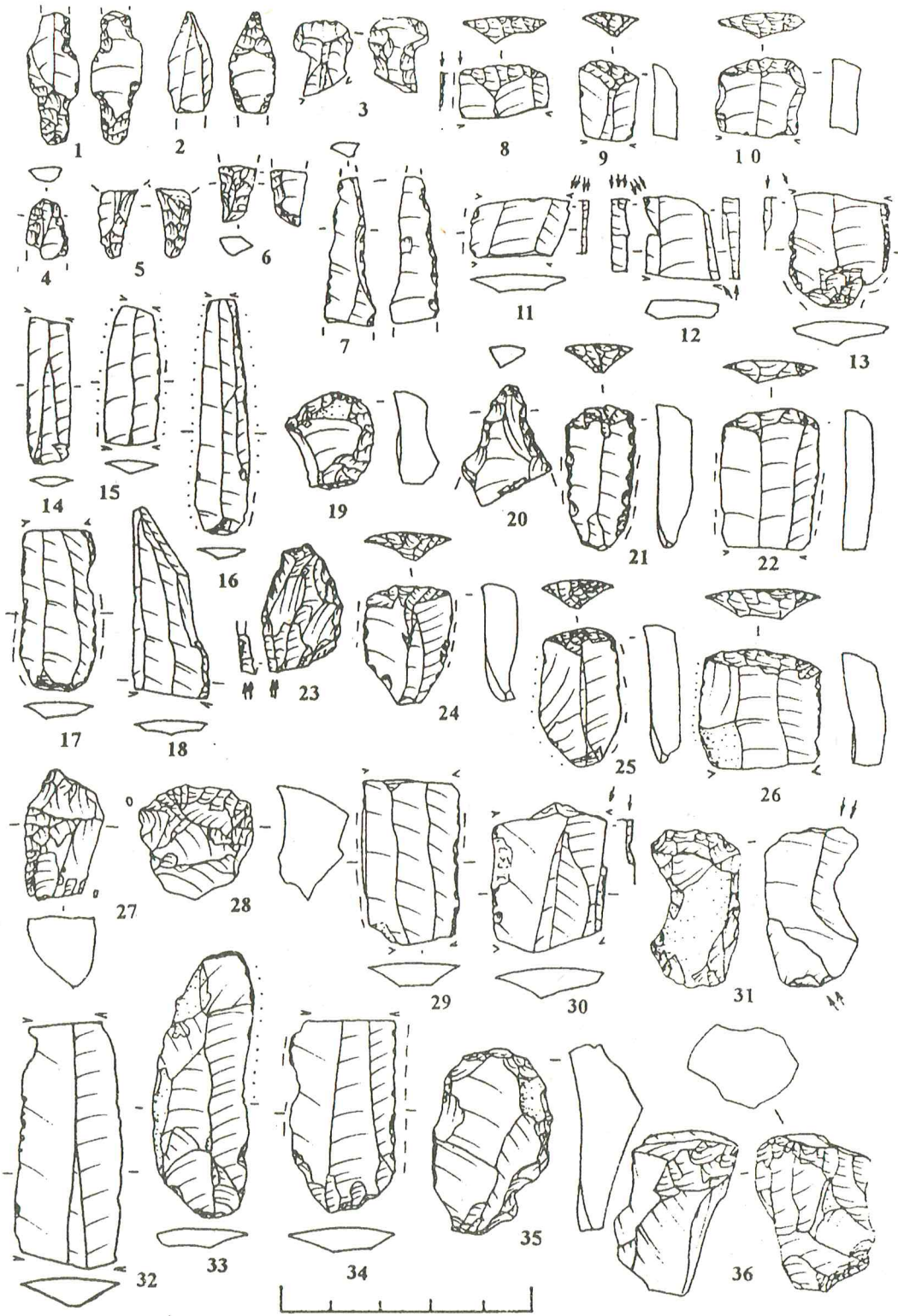
7 pav. Drenių radimvietės ankstyvojo mezolito titnago dirbiniai
