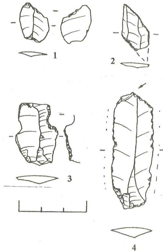
10 pav. Spigino salos mezolito kapų titnago inventoriųs
